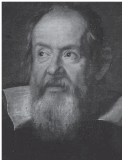
伽利略
